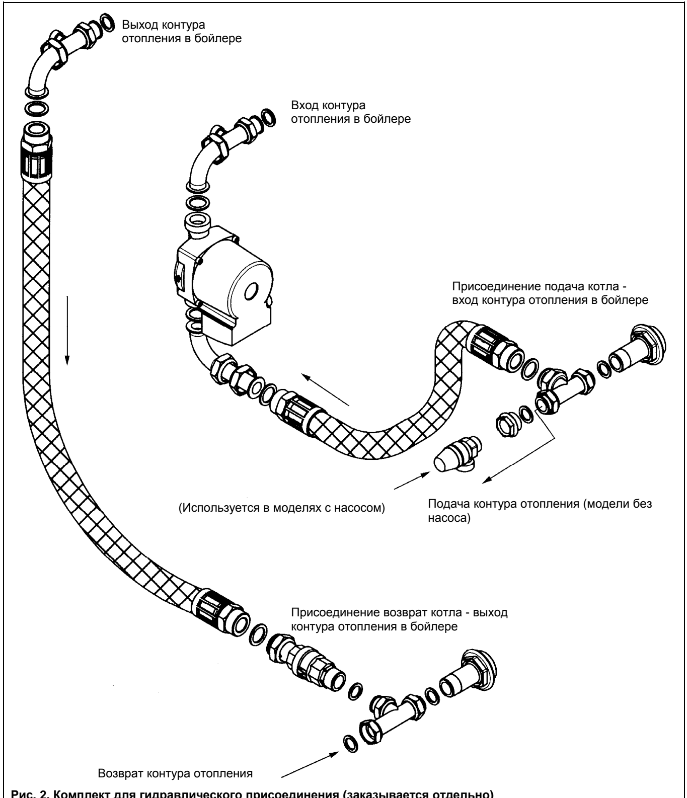
Рис. 2. Комплект для гидравлического присоединения (заказывается отдельно)
